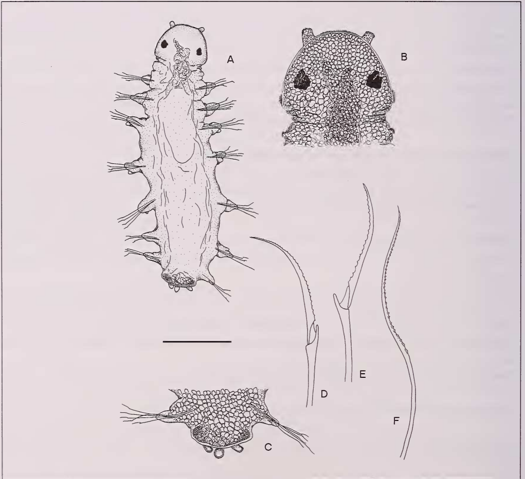
Figura 2. Lacydonia miranda .- A: Aspecto general, visión dorsal; B: Prostomio; C: Pigidio; D: Seda compuesta del cuarto setífero.
